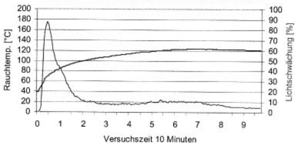
#1897 Verseidag,PVC-besch.Polyesterg.B1104,unbedruckt, Kette Restlänge: 60 cm, Rauchtemp.:123°C, Rauch-Int.: 138%min
